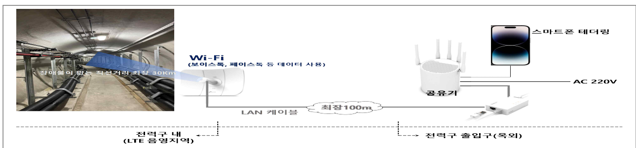
[그림 1] 지하전력구 내, 외부통신망 구성도
